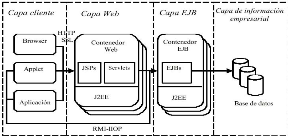
Arquitectura global del sistema
