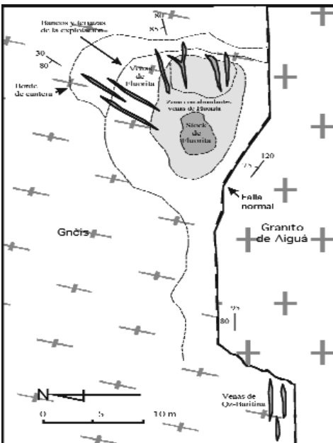
Figura 1. Esquema geológico en planta de la mineralización y labores de Mina Florencia. Modificado de Bosse et al. (1982).
