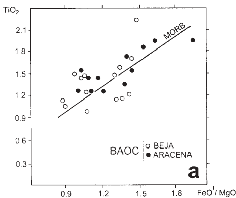
Fig. 4.a - Diagrama de projecção do TiO_2 versus FeO^{(0)}/MgO para as litologias do COBA. A linha a cheio representa os basaltos com características MORB. Os círculos a negro representam as rochas máficas do segmento de Aracena do COBA (DUPUY et al. , 1979); os círculos a branco representam as rochas máficas do segmento de Serpa-Beja do COBA (QUESADA et al. , 1994). b - Gráficos de comparação aos condritos normalizados dos elementos incompatíveis em rochas máficas do COBA, MORB e IAB (i.e., 'mid-ocean ridge basalts' e 'island arc basalts') — segundo QUESADA et al. (1994).
