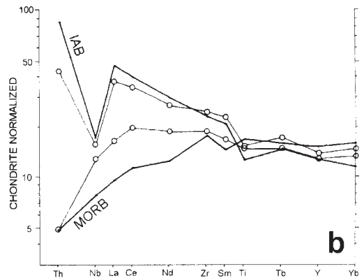
Fig. 4.a - Diagrama de projecção do TiO_2 versus FeO^{(0)}/MgO para as litologias do COBA. A linha a cheio representa os basaltos com características MORB. Os círculos a negro representam as rochas máficas do segmento de Aracena do COBA (DUPUY et al. , 1979); os círculos a branco representam as rochas máficas do segmento de Serpa-Beja do COBA (QUESADA et al. , 1994). b - Gráficos de comparação aos condritos normalizados dos elementos incompatíveis em rochas máficas do COBA, MORB e IAB (i.e., 'mid-ocean ridge basalts' e 'island arc basalts') — segundo QUESADA et al. (1994).
