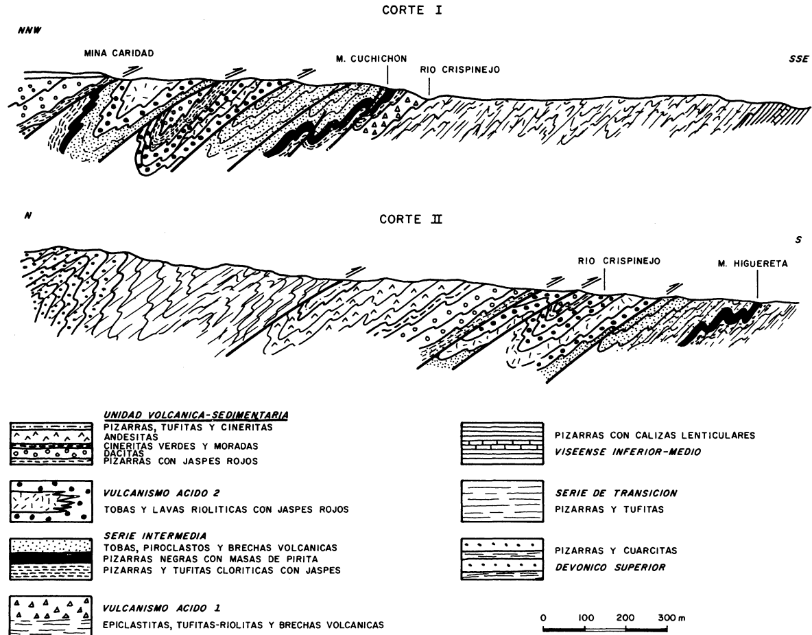
Figura 2.- Cortes geológicos de la estructura sinclinal de Aznalcollar.
