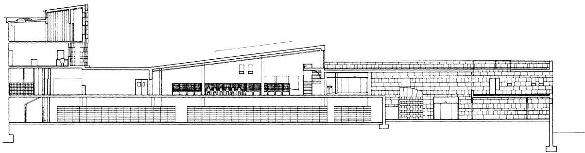
SECCION 4
