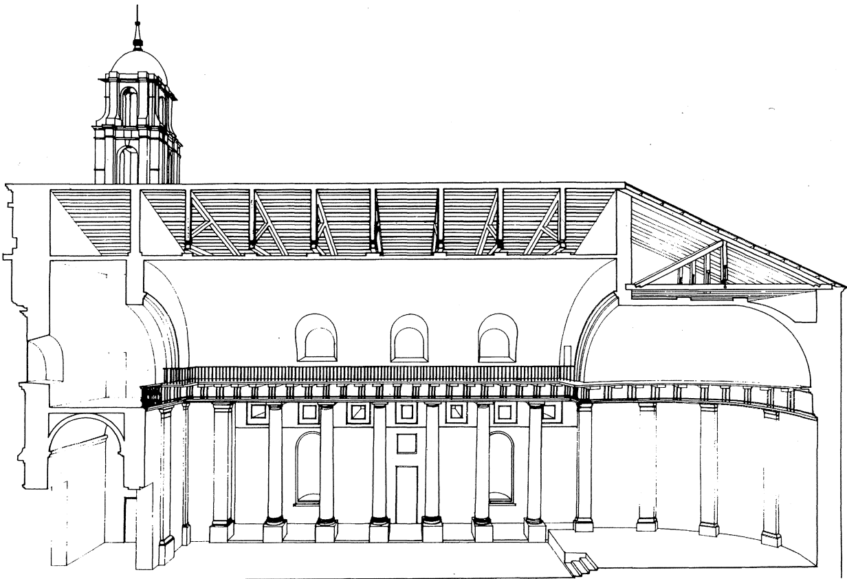
PERSPECTIVA INTERIOR SECCIONADA
