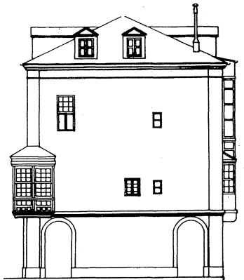
ALZADO LATERAL
