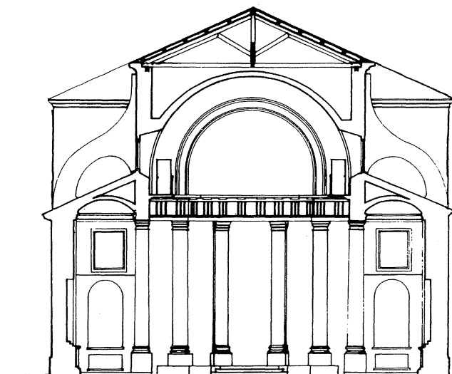
SECCION TRANSVERSAL
