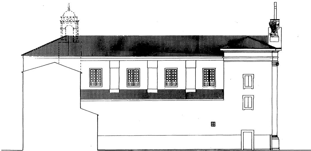
ALZADO CALLEJON LATERAL
