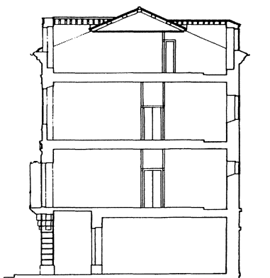
SECCION
