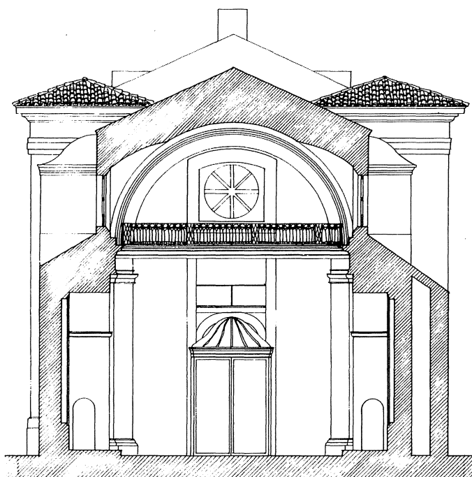
SECCION TRANSVERSAL
