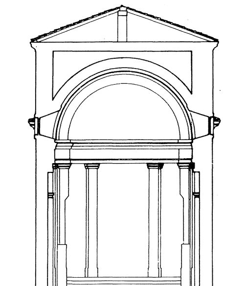
SECCION TRANSVERSAL
