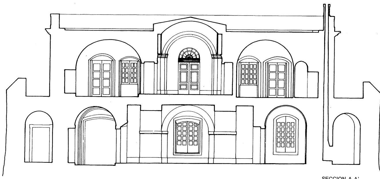
SECCION A-A'
