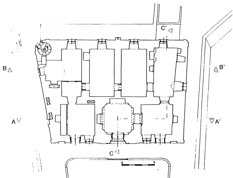
PLANTA
