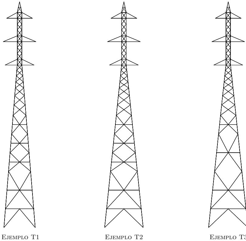
Figura 10: Ejemplos T1, T2 y T3. Comparación entre los diseños finales obtenidos.
