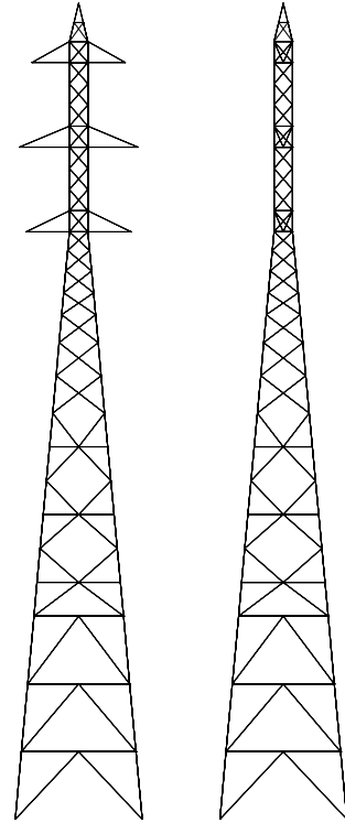
Figura 6: Torre de alta tensión tipo FECSA/GL-110KV (frente y perfil).
