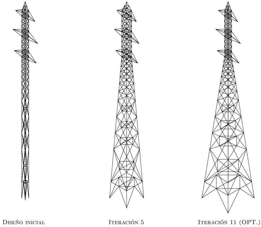
Figura 9: Ejemplo S2. Evolución del diseño estructural
