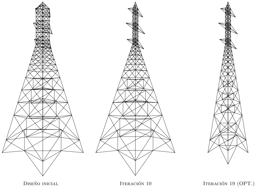
Figura 8: Ejemplo S1. Evolución del diseño estructural
