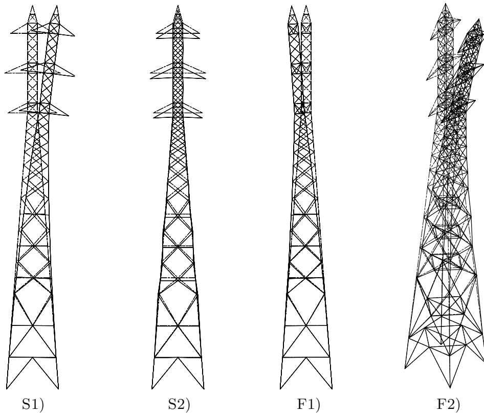
Figura 7: Hipótesis de carga tipificadas (de izquierda a derecha): S1) carga de viento; S2) carga de hielo; F1) disequilibrio de tracciones; F2) rotura de un cable conductor.
