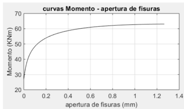
Figura 7. Diagramas momento-apertura de Fisura para las secciones de solera de proyecto.
