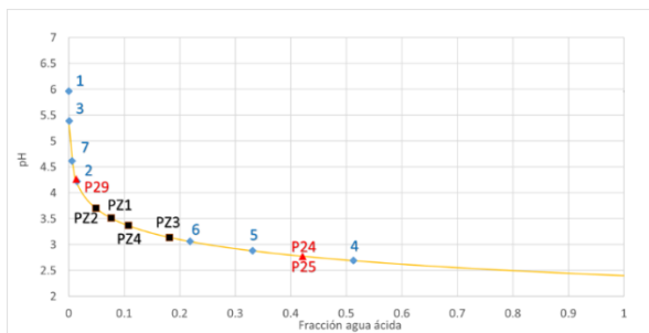
Fig. 10. Fracción de agua ácida y valor medio del pH medido en los 7 puntos de seguimiento de la calidad del agua en aguas superficiales y en los 7 piezómetros situados en el terraplén del Aparral (ver Fig. 2), presentado sobre la línea de mezcla de un agua ácida con un pH 2,4 y un agua natural con un pH de 5,4.
