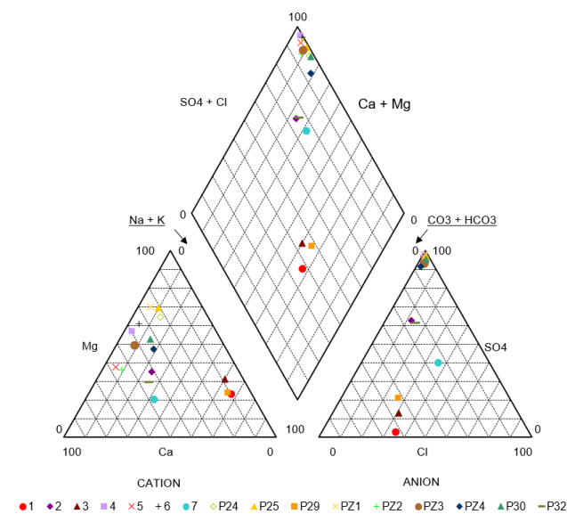
Fig. 9. Diagrama de Piper de las muestras tomadas en septiembre de 2020 en los 7 puntos de seguimiento de la calidad del agua superficial (ver Fig. 2) y las muestras de los piezómetros de la red de control.
