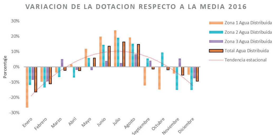
Figura 4 | Variación de la dotación mensual en las distintas zonas del sistema.
