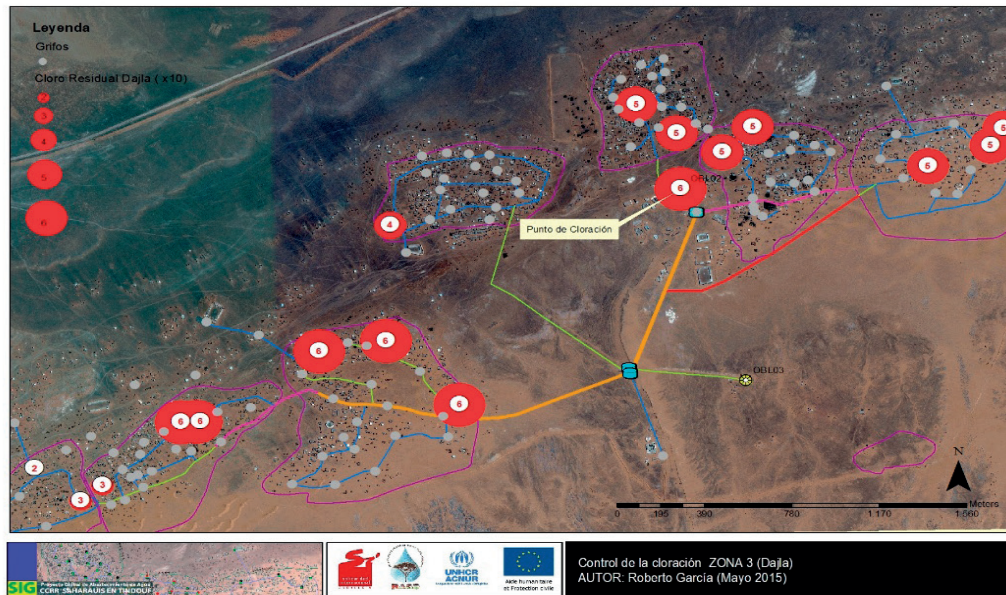
Figura 5 | Estudio control de la cloración red de agua en Dajla (Zona III). Se presentan, sobre una imagen satélite de la zona, las concentraciones medidas de cloro residual (en ppm×10) en puntos significativos de la red de abastecimiento previamente definidos en el protocolo de calidad del agua del PSA-CRS. Se muestran también los elementos principales de la red - el pozo (círculo amarillo), depósitos, grifos y tuberías de diferente tamaño (líneas de colores)- y los diferentes sectores en que se divide la red de distribución, que se corresponde con divisiones administrativas llamadas Dairas (delimitados con polígonos rosas).
