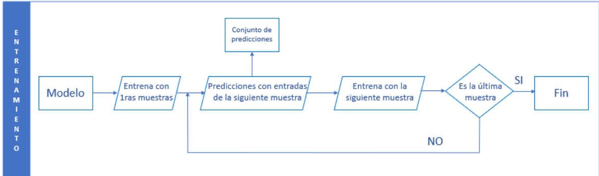
Figura 19: Diagrama de flujo da metodoloxía Walk Forward Validation
