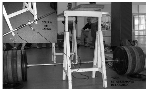
FIGURA 1. Barra olímpica con una carga de 210 kgs. y estabilizada con dos discos en cada extremo. La célula de carga se fija en el medio de la barra con un mosquetón.
