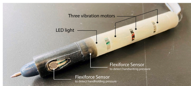
Fig. 29. ApEn: the stress-aware pen.
