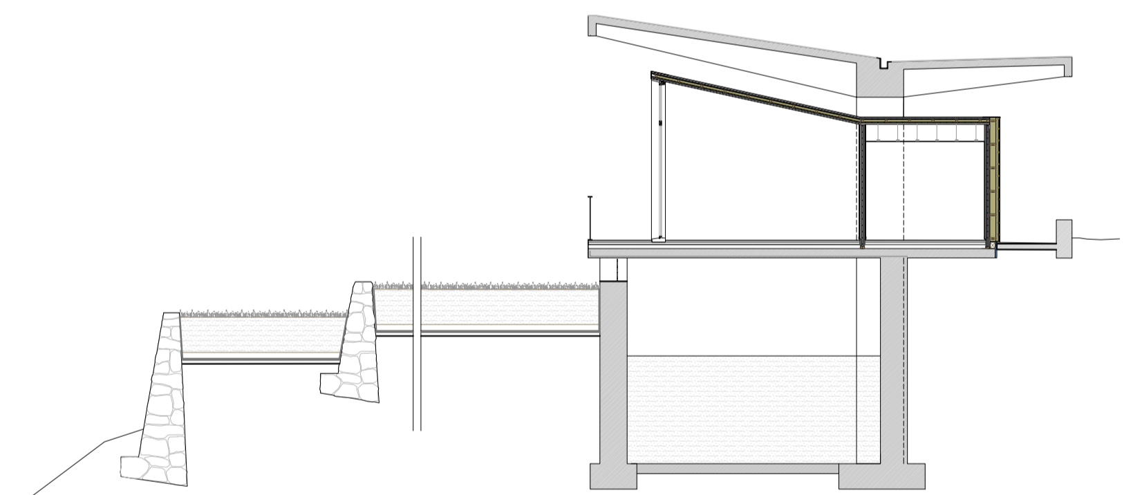
SECCIÓN CO-WORKING
