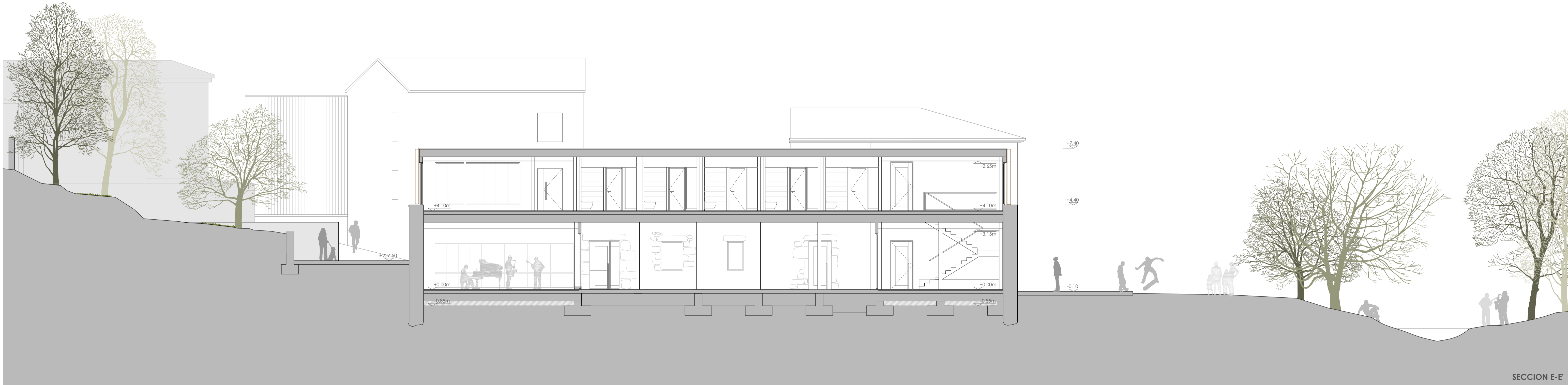
SECCION E-E'
