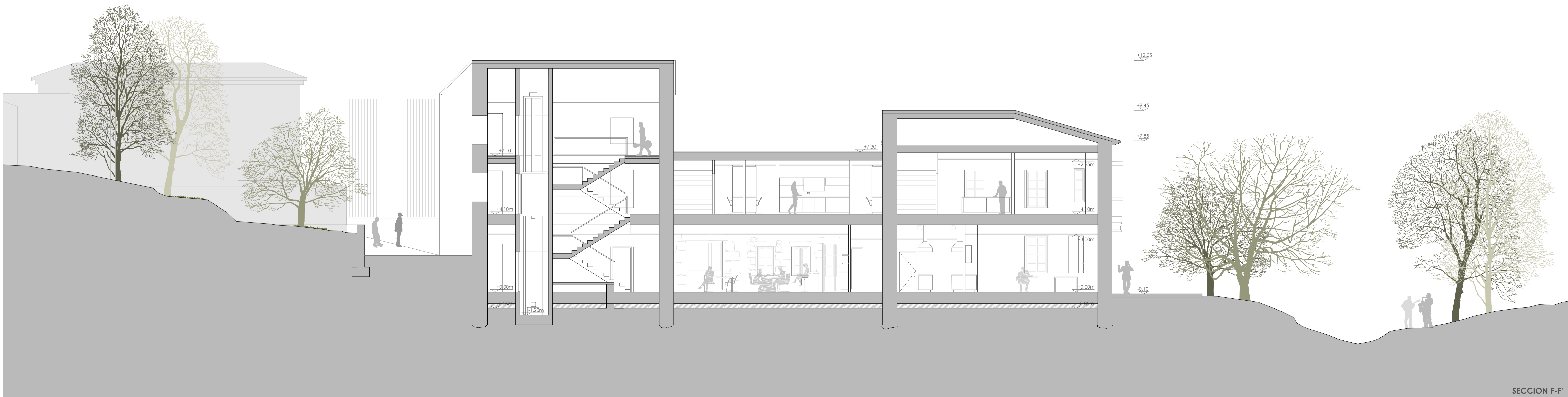
SECCION F-F'
