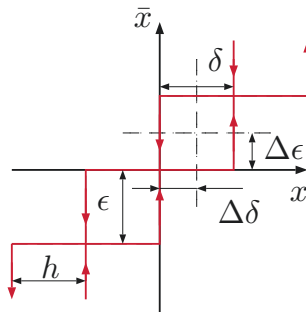
Figura 2: Relación entrada-salida del muestreo SSOD.
