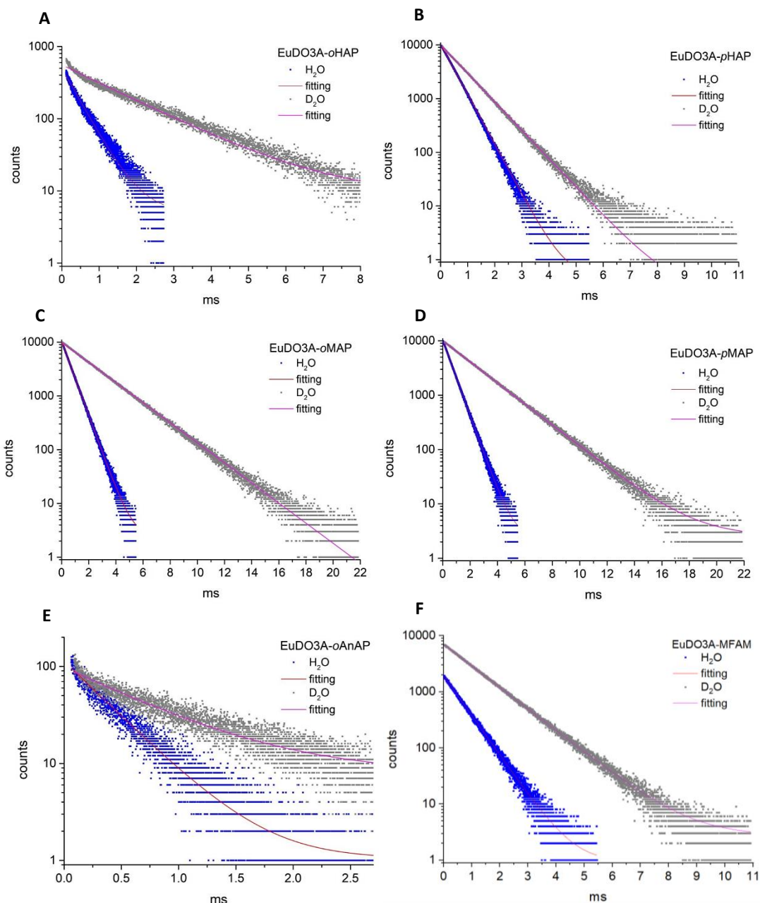
Figura 36: Curvas de decaemento e axuste exponencial en H 2 O e D 2 O dos complexos estudados ( \lambda_{em} = 613 nm). A) EuDO3A- o -HAP (pH 4,9; \lambda_{exc} = 350 nm). B) EuDO3A- p -HAP (pH 5,1; \lambda_{exc} = 314 nm). C) EuDO3A- o -MAP (pH 7,4; \lambda_{exc} = 350 nm). D) EuDO3A- p -MAP (pH 7,4; \lambda_{exc} = 310 nm). E) EuDO3A- o -AnAP (pH 7,4; \lambda_{exc} = 400 nm). F) EuDO3A-MFAM (pH 6,3; \lambda_{exc} = 319 nm).
