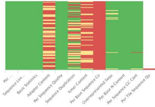
Figura 3. Resultados de los análisis de calidad. Cada columna representa un parámetro de calidad, mientras que cada barra es cada una de las muestras. Una barra en verde significa que esa muestra está por encima del umbral de calidad para ese parámetro, en amarillo está en este umbral y en rojo por debajo de este
