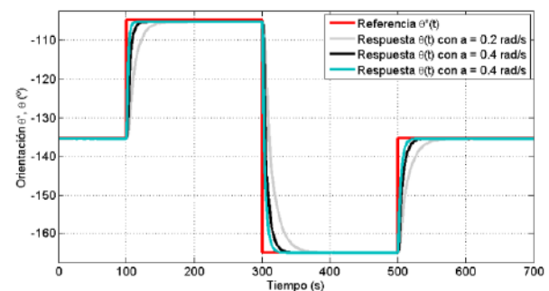
Figura 8.b. Respuestas temporales de la orientación \theta(t)
