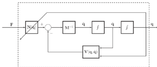
Figura 5: Modelo dinámico propuesto para el diseño del controlador
