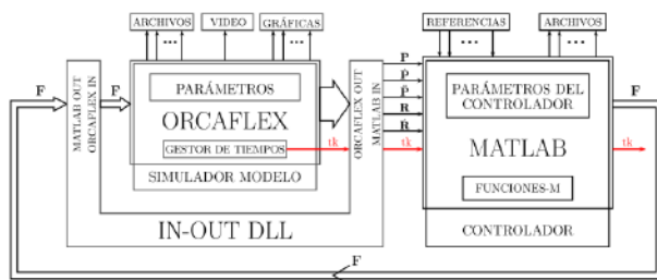
Figura 7. Sistema de Integración Matlab-OrcaFlex
