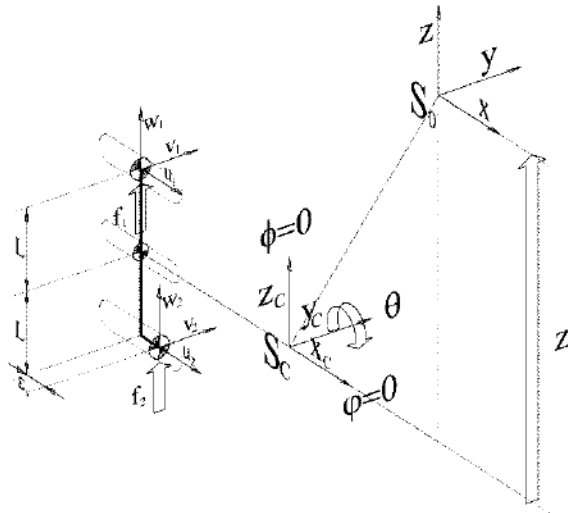
Figura 4: Sistemas de referencia y variables
