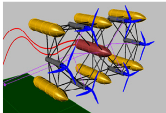
Figura 2: Perspectiva del generador multi-rotor.
