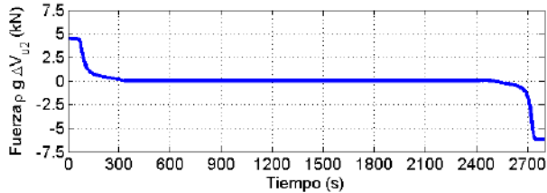
Figura 11. Fuerzas aplicadas por los flotadores durante la realización de la maniobra de cambio de orientación
