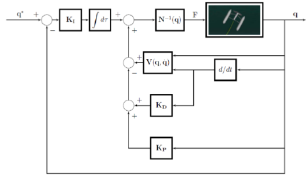
Figura 6. Sistema de control multivariable no lineal.
