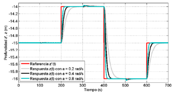
Figura 8.a. Respuestas temporales de la profundidad z(t)
