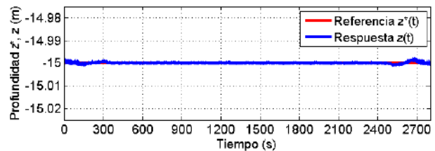
Figura 9. Respuesta temporal de la profundidad, durante la realización de la maniobra de cambio de orientación
