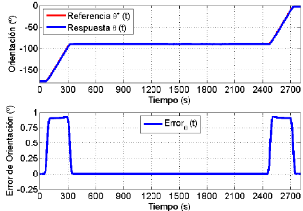
Figura 10. Respuesta temporal del ángulo, durante la realización de la maniobra de cambio de orientación.
