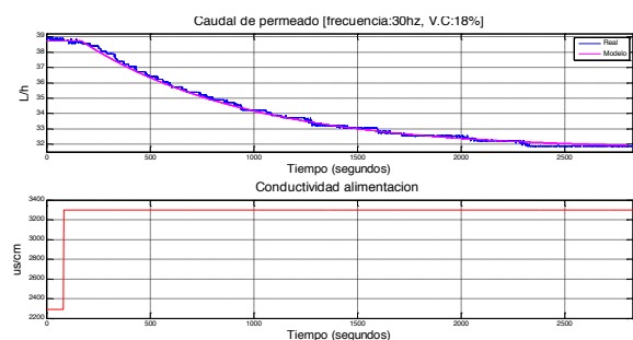
Figura 4: Respuesta del caudal de permeado frente a un cambio de la CE del agua de alimentación.
