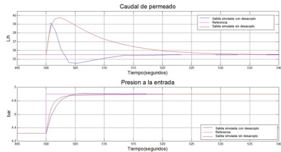
Figura 6: Efecto sobre el caudal de un cambio de consigna en la presión son y sin desacoplo.
