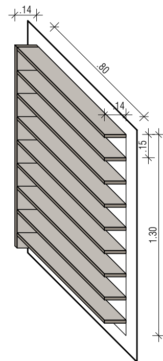
Ventana cocina ESC.: 1/25
