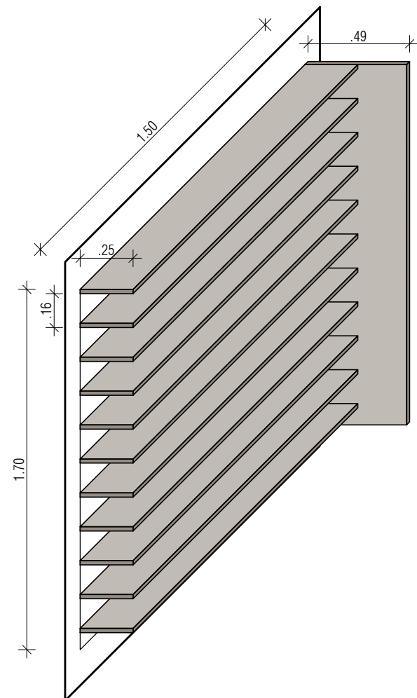
Ventana habitación ESC.: 1/25
