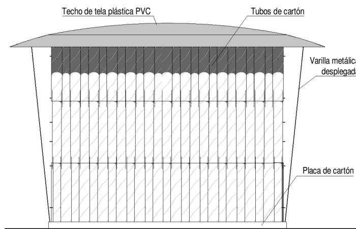
Alzado 04
