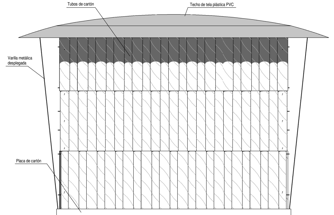
Alzado 02
