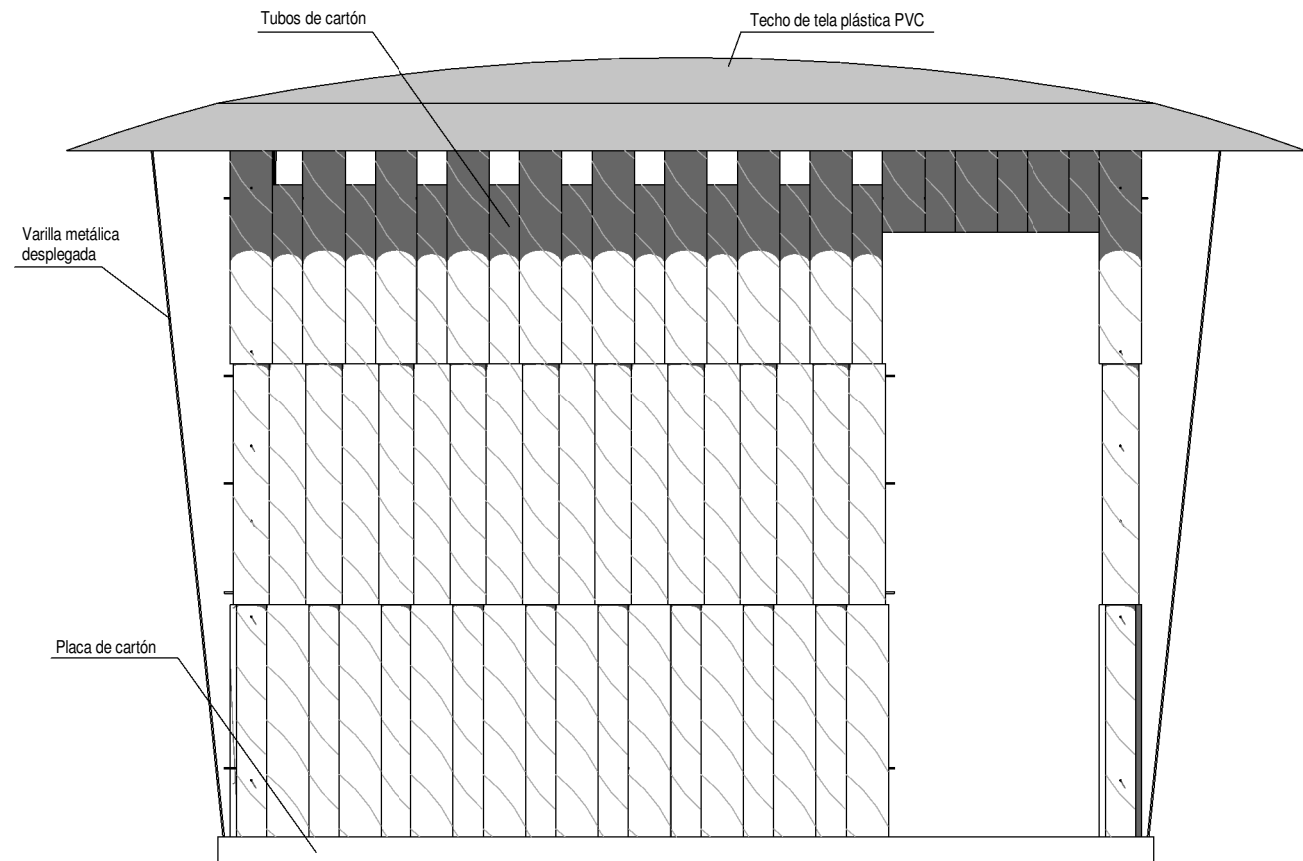
Alzado 01
