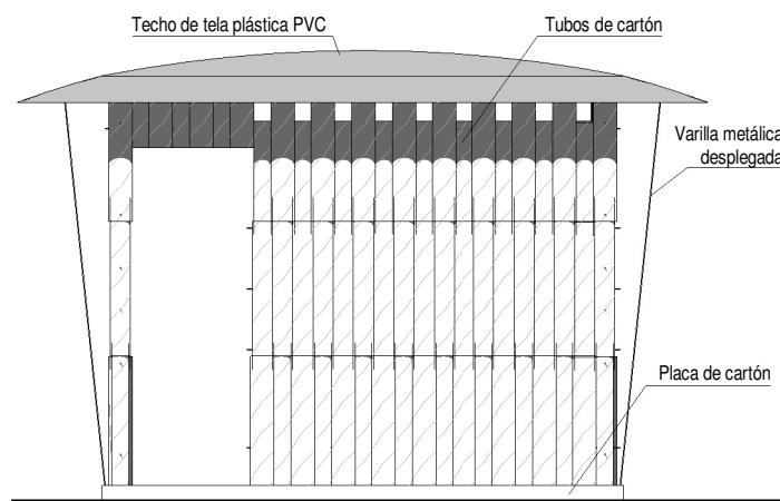
Alzado 03
