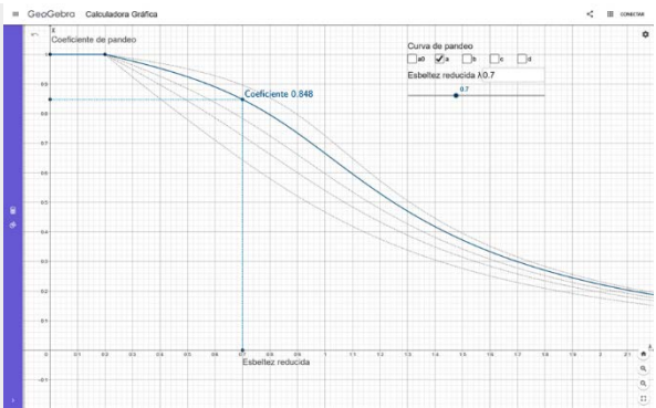
Figura 6. Análisis de las curvas europeas de pandeo mediante Geogebra
