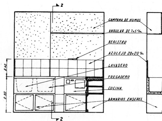
Figura 5: Alzado y sección cocina tipo INV Fuente: Hogar y Arquitectura , n.º 2 (1956)
