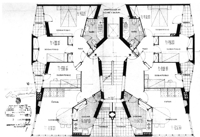
Figura 3: José Antonio Coderch, La Barceloneta (1951), Barcelona Fuente: Archivo Histórico COAC Barcelona
