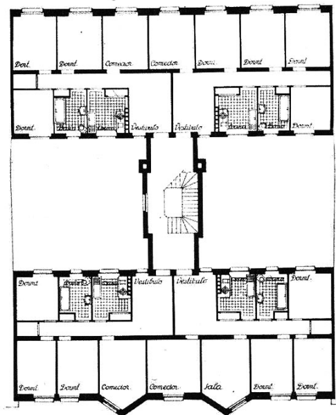
Figura 1: Secundino Zuazo, Casa de las Flores (1931), Madrid Fuente: Arquitectura , n.º 1 (enero 1933)
