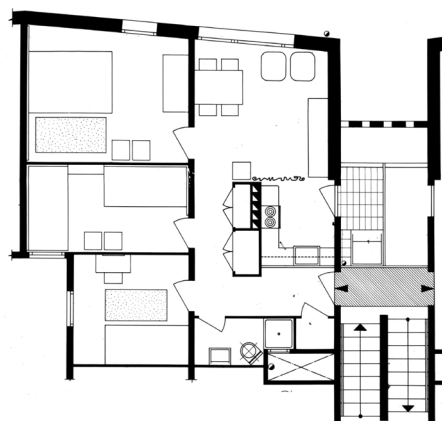
Figura 6: Josep Maríà Martorell y Oriol Bohigas, Pallars (1955), Barcelona Fuente: Cuadernos de Arquitectura , n.º 44 (1961)
