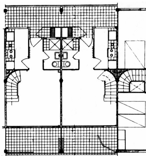
Figura 2: Josep Lluís Sert, Casa Bloc (1932), Barcelona Fuente: AC. Documentos de Actividad Contemporánea (1933)
