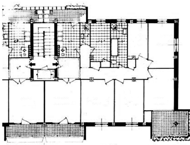
Figura 4: Rodolfo García de Pablos y Manuel Manzano-Monís, Colonia Nta. Sra. de Montserrat (1953), Madrid Fuente: M a . Antonia Fdez. Nieto (2006)
