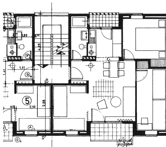
Figura 7: Luis Gutiérrez Soto, Gran San Blas (1958), Madrid Fuente: COAM. La obra de Luis Gutiérrez Soto (1978)
