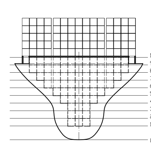
Cubierta 17 – Columna A/B 150 TEU's Bodega 17 – Columna A/B 134 TEU's
