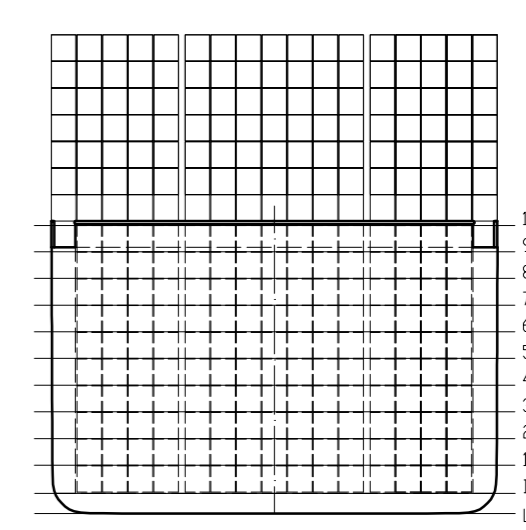
Cubierta 11 – Columna A/B 238 TEU's Bodega 11 – Columna A/B 300 TEU's
