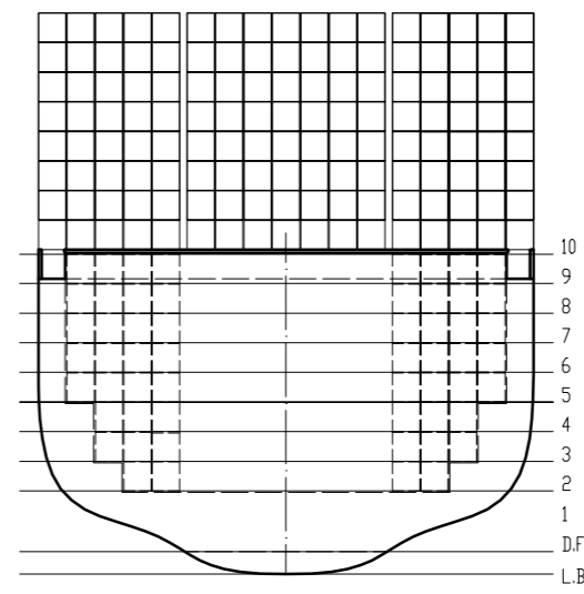
Cubierta 4 – Columna B 216 TEU's Bodega 4 – Columna A/B 224 TEU's
