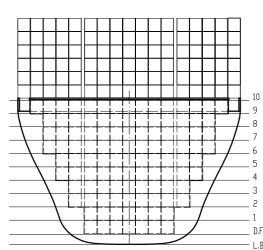
Cubierta 15 – Columna A/B 204 TEU's Bodega 15 – Columna A/B 216 TEU's
