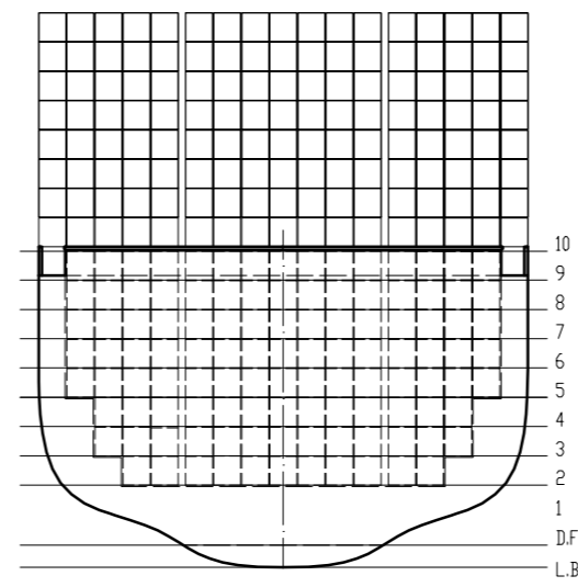
Cubierta 4 – Columna A 272 TEU's Bodega 4 – Columna A/B 224 TEU's
