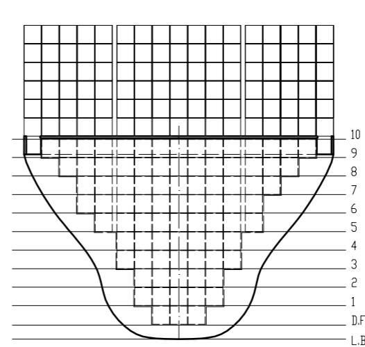
Cubierta 16 – Columna A/B 204 TEU's Bodega 16 – Columna A/B 172 TEU's
