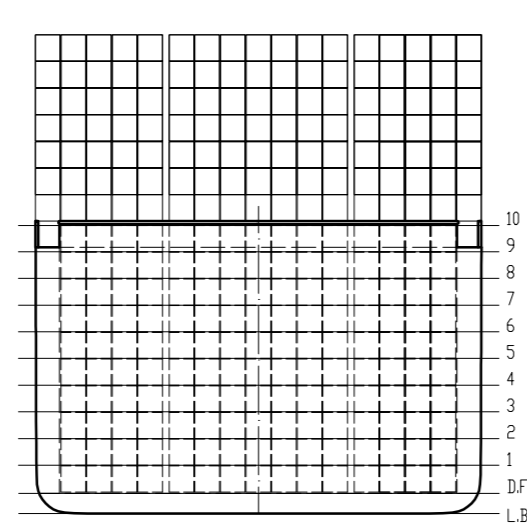
Cubierta 7 – Columna A/B 238 TEU's Bodega 7 – Columna A/B 300 TEU's
