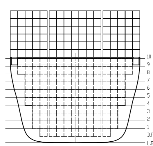
Cubierta 14 – Columna A/B 204 TEU's Bodega 14 – Columna A/B 248 TEU's
