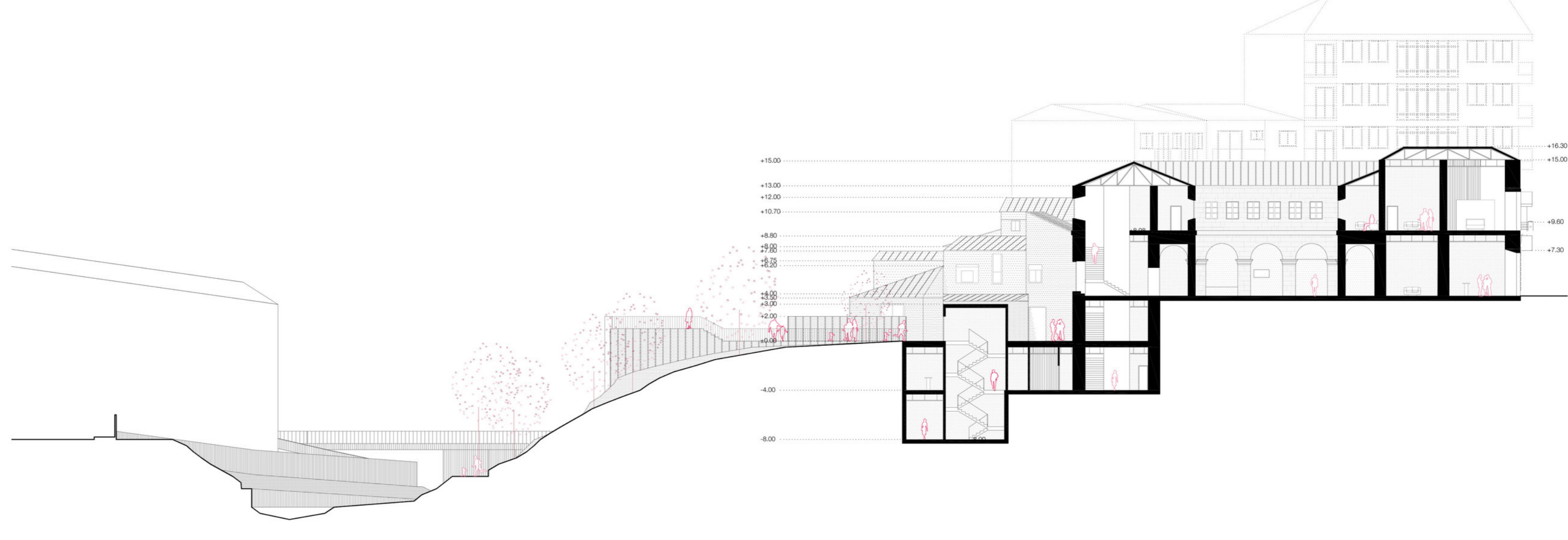
SECCIÓN TRANSVERSAL HOTEL
