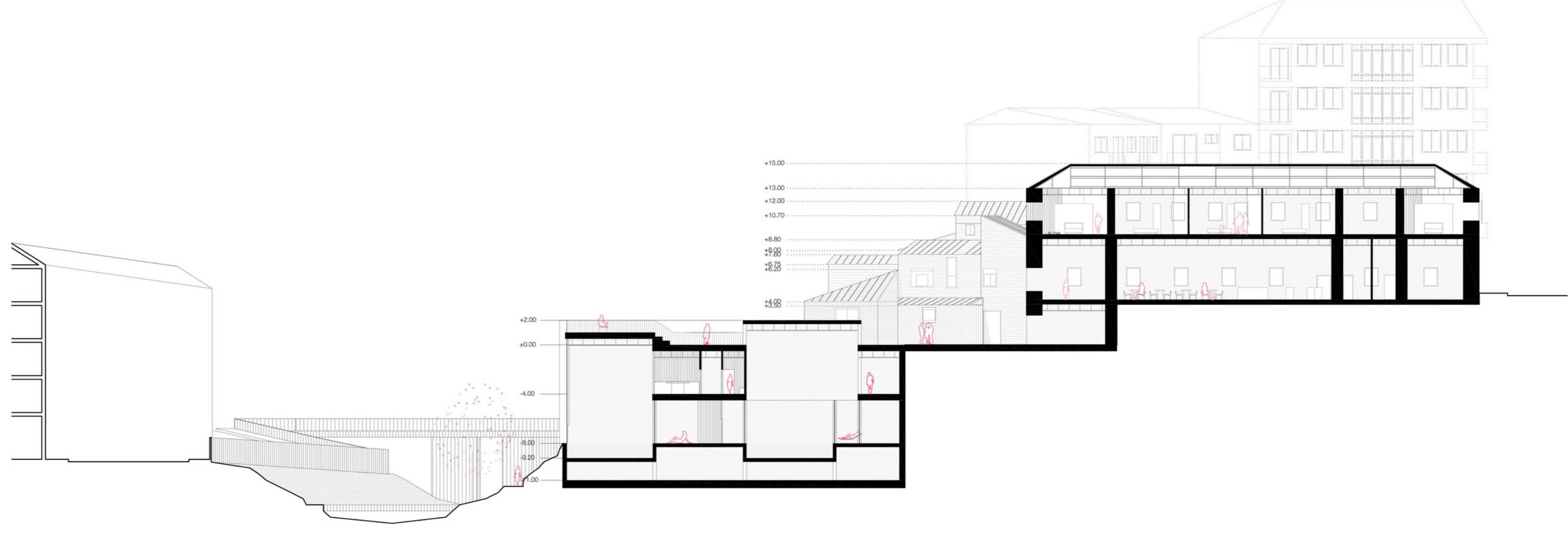
SECCIÓN TRANSVERSAL BALNEARIO Y HOTEL
