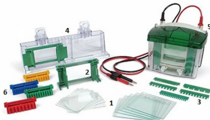
Figura 8. Equipo de western-blot. 1- Cristales para el molde, con espaciadores integrados; 2- Marco, soporte para los cristales; 3- Peines con diferente número de pocillos; 4- Soporte del marco; 5- Tanque de tampón; 6- Guía para el cargado de las muestras. Imagen de representativa extraída de la web de Bio Rad (Hercules, California, EE.UU.).
