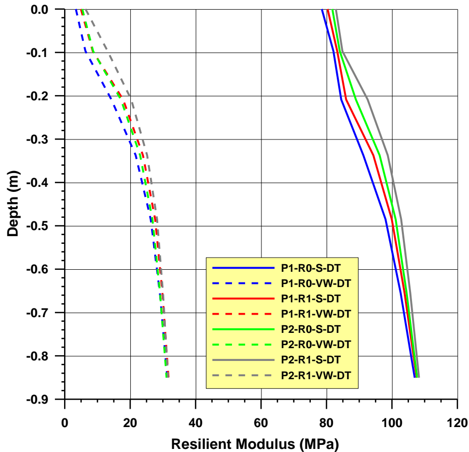
Figura. 2. Módulo resiliente en la explanada (explanada S and VW, DT).
