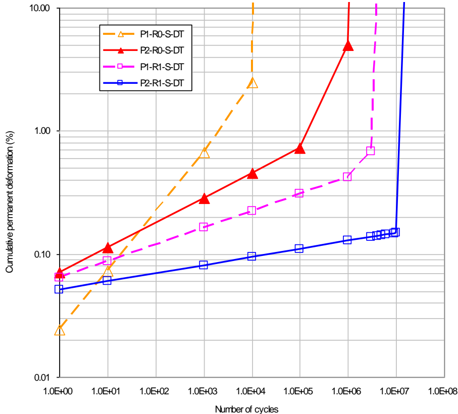
Figura 5. DP acumulada en la capa de reciclado (explanada resistente)
