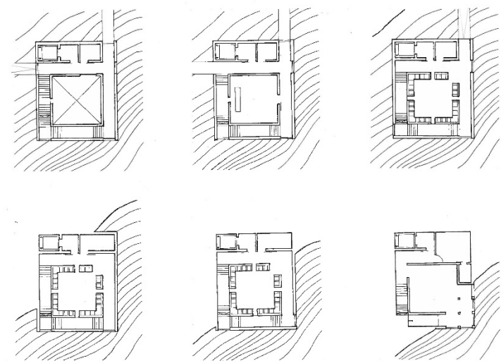
OTERO PEREZ ALBERTO PLANTAS E:1:200
