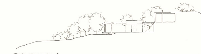
SECCIÓN TRANSVERSAL 2
