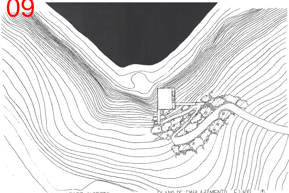
OTERO PEREZ ALBERTO PLANO DE EMPLAZAMIENTO E:1:400
