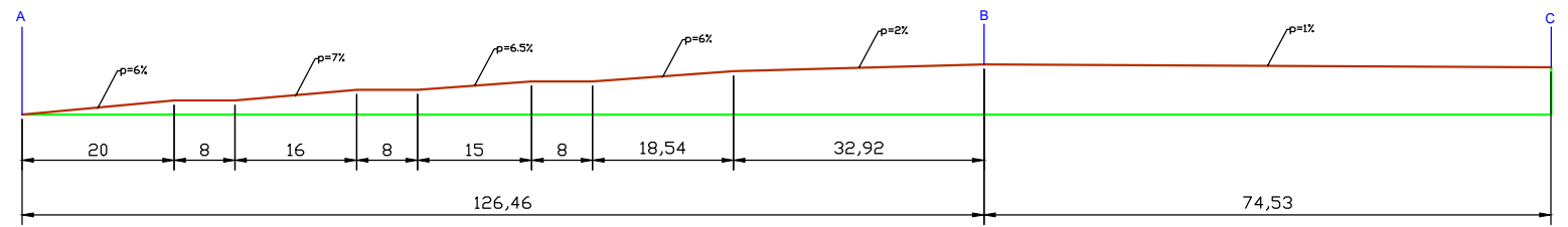
Desarrollo longitudinal de A a C Escala 1:1000
