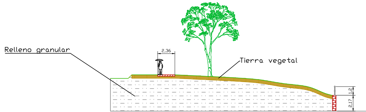
SECCIÓN A-A' Escala 1:250
