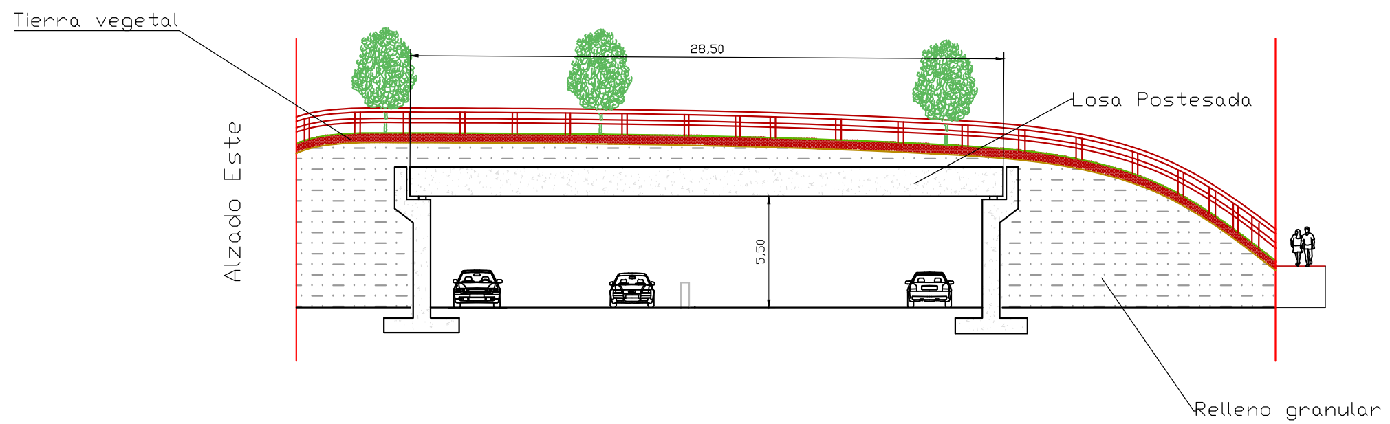
SECCIÓN TIPO LOSA Escala 1:250
