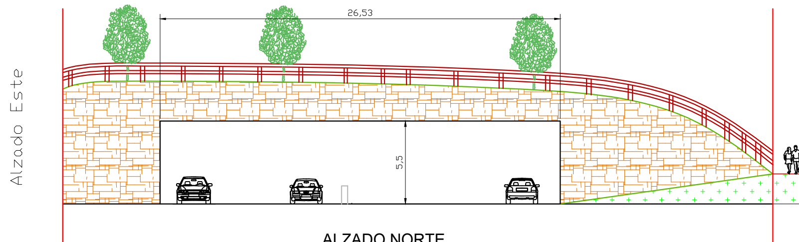
ALZADO NORTE Escala 1:250
