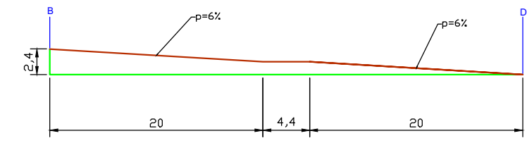
Desarrollo longitudinal de B a D Escala 1:500
