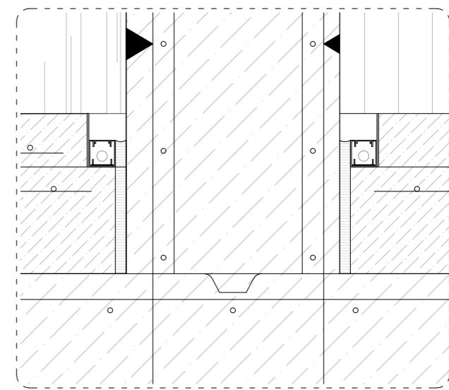
detalle caja leds a pie e muro 1/10
