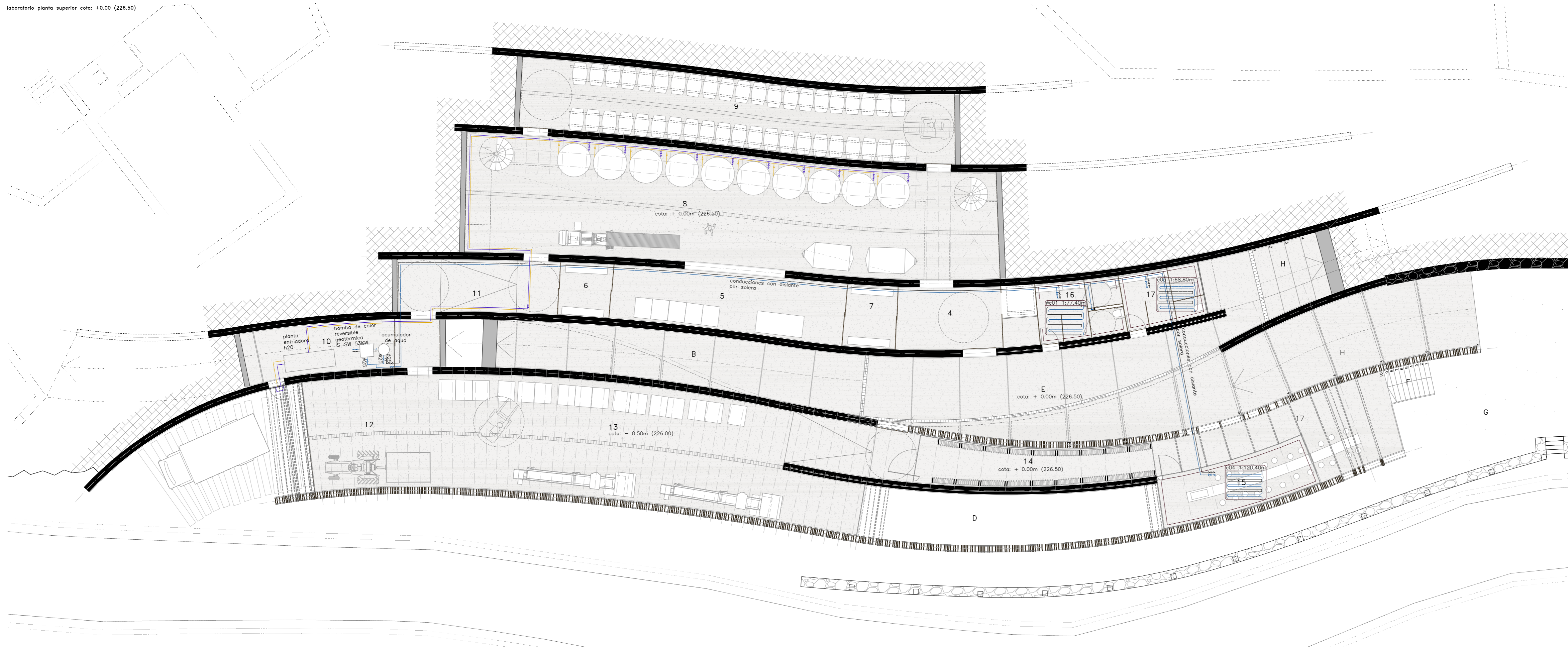
1. VESTIBULO SUPERIOR 2. LABORATORIOS 3. PASADIZO SOBRE CUBAS 4. VESTIBULO INFERIOR 5. ZONA DE ALMACENAJE GENERAL 6. TALLER MANTENIMIENTO 1 7. TALLER MANTENIMIENTO 2 8. ZONA DE ELABORACION Y CUBAS DE ACERO 9. ZONA ALMACENAJE EN BARRICA 10. CENTRAL DE FRIO E INSTALACIONES 11. RAMPA Y ZONA DE PASO 12. GARAJES MAQUINARIA Y COCHES 13. DISTRIBUCION Y EMBOTELLADO 14. CAVA DE VINOS 15. SALA DE CATAS 16. ASEOS COMUNES 17. VESTUARIOS PERSONAL A. PASEO SUPERIOR B. RAMPA ACCESO C. HALL SUPERIOR D. PATIO E. ESPACIO SEMIEXTERIOR F. ESCALERAS EXTERIORES G. VIÑAS H. RAMPA ESCALONADA
