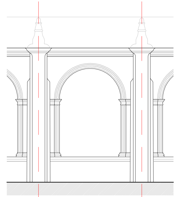
ALZADO MODIFICACIÓN
