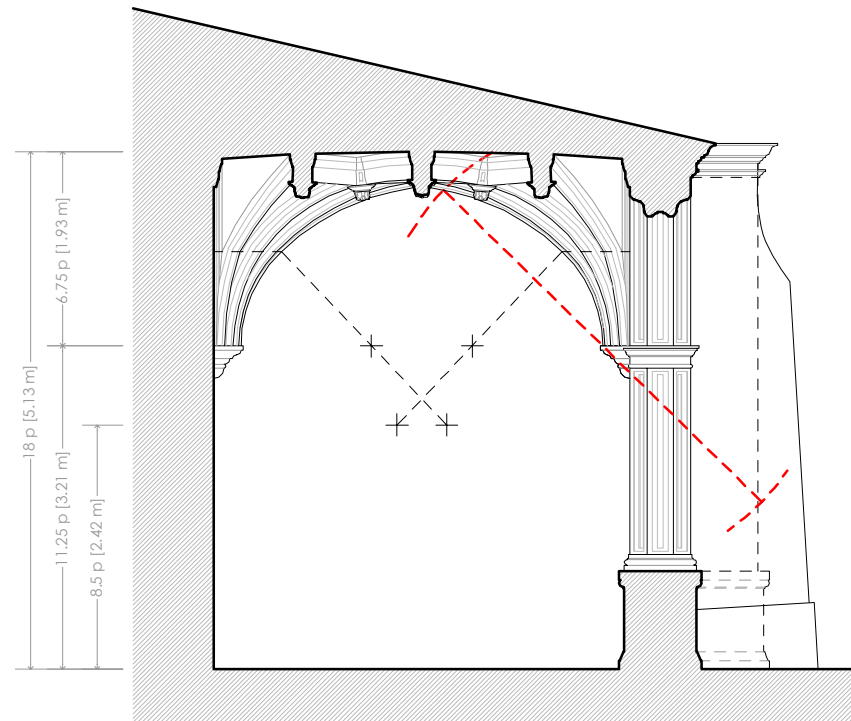
RELACIÓN SECCIÓN CONTAFUERTES PROYECTO-MODIFICACIÓN
