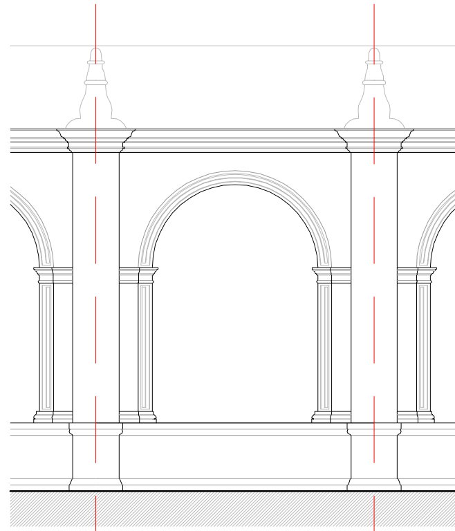
ALZADO PROYECTO (HIPÓTESIS)
