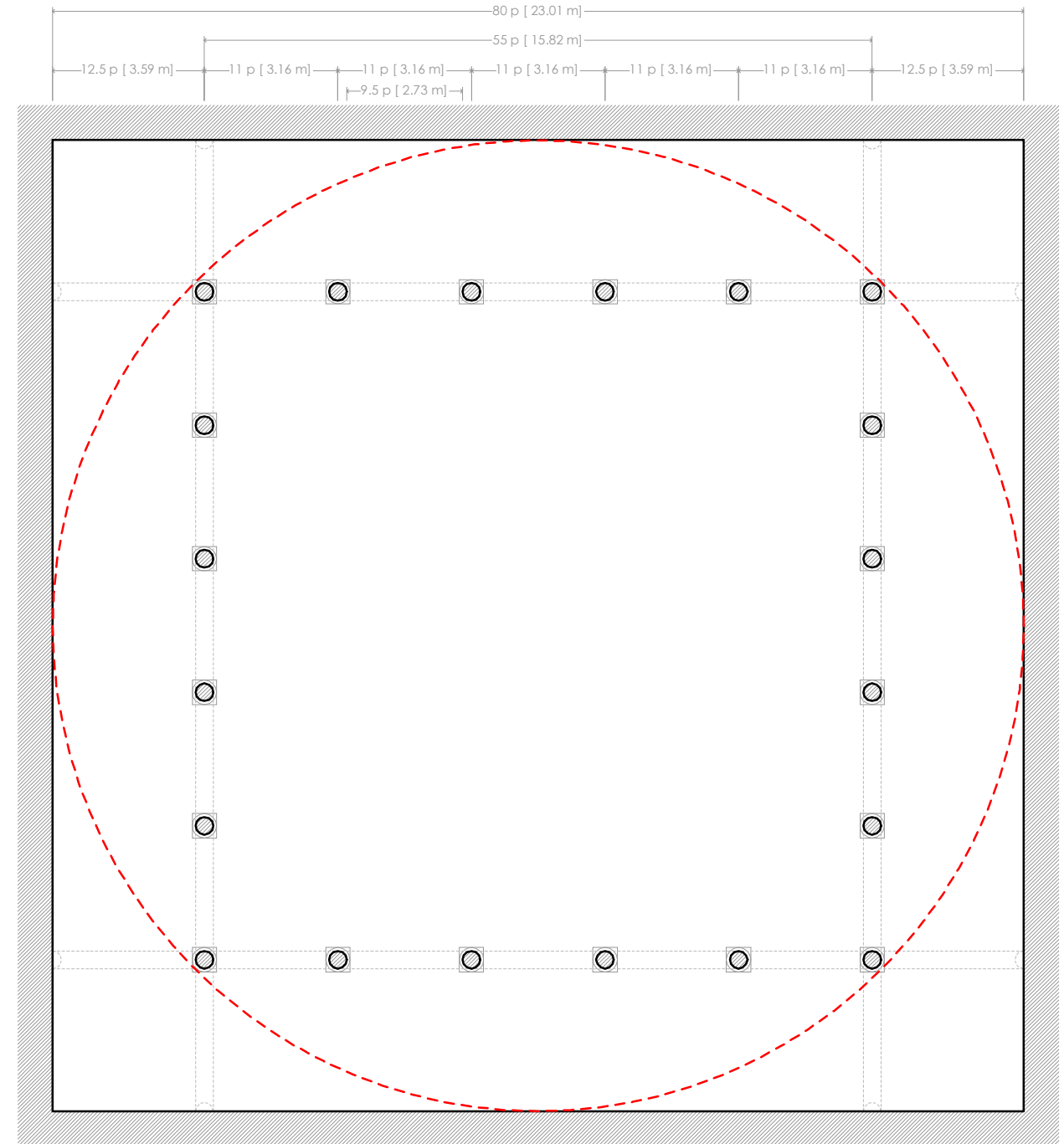
RECONSTRUCCIÓN PLANTA CLAUSTRO PÚBLICO
