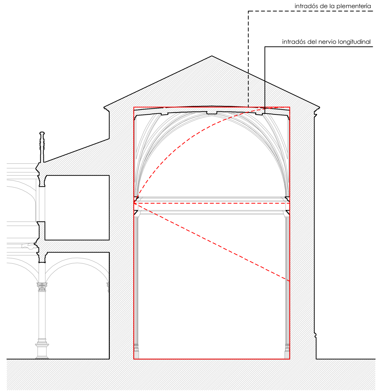
sección transversal -Capilla-
