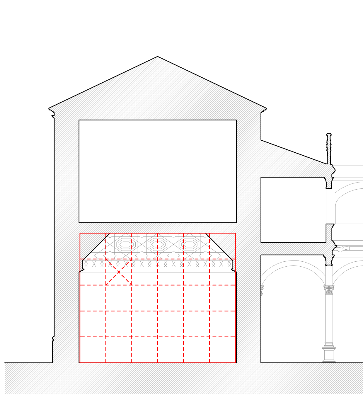
sección transversal -General de Teología-
