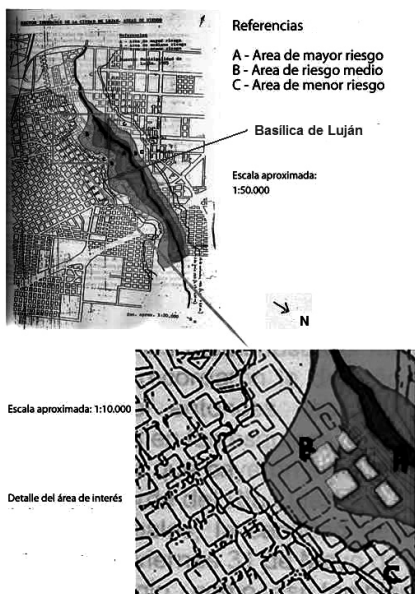
Fig. 11 y 12. La gran última inundación del año 1985 de la ciudad de Luján. En los mapas se observa el alcance de las áreas de riesgo y en la fotografía el impacto sobre la Basílica de Luján, en que el agua alcanzó los 6.40 mts. de altitud. Fuentes: Cartografía adaptada de C. Haas (1995) y fotografía de R. Varela, LAB VARELA, 1985.
