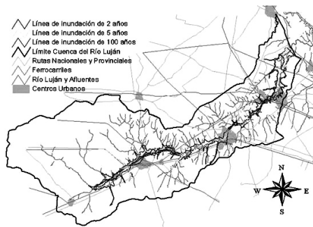
Fig. 9. Períodos de recurrencia de inundaciones en la cuenca del río Luján de la Provincia de Buenos Aires; apud Chiozza y otros, 2009.
