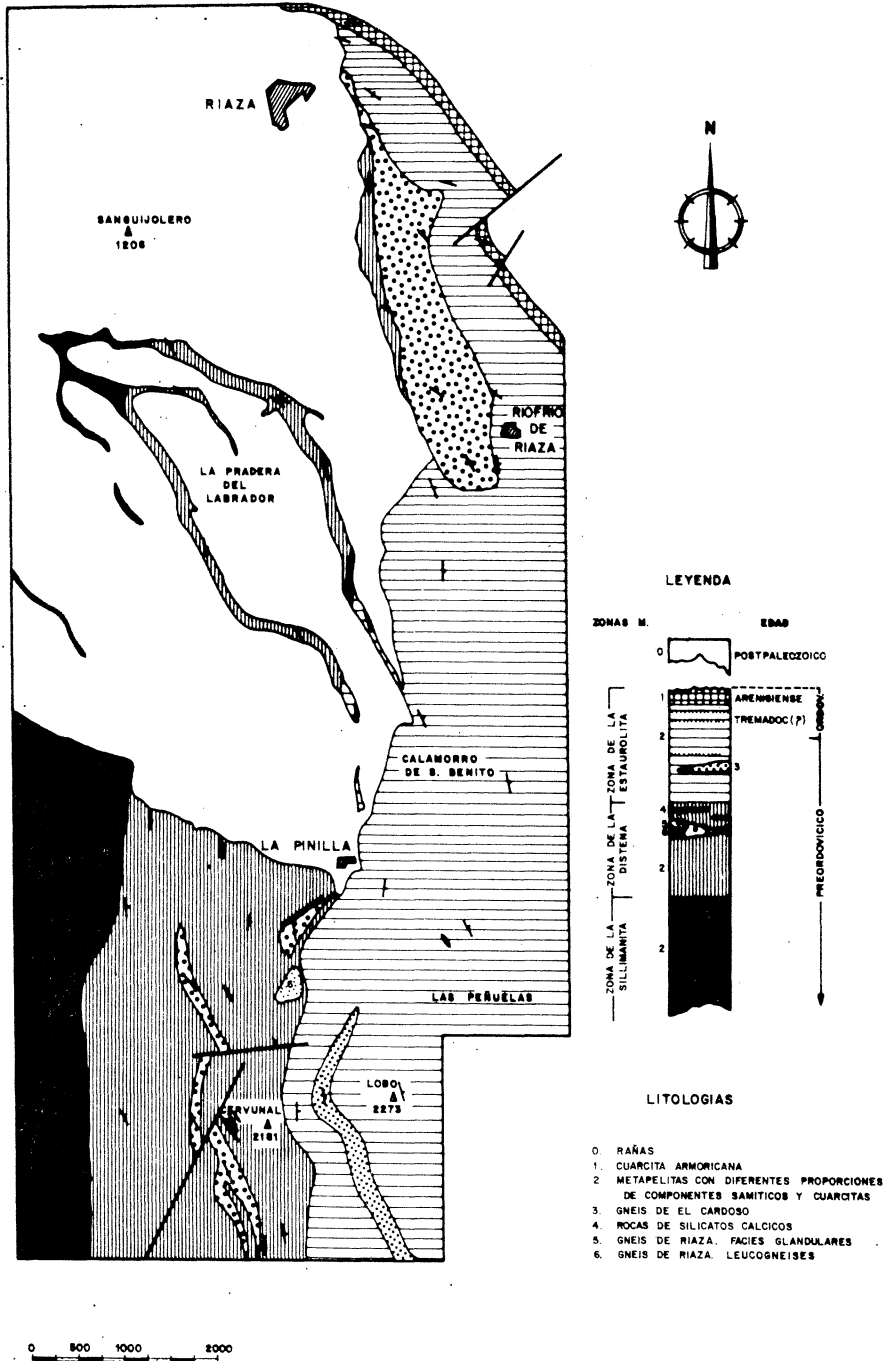
Fig. 2.—Mapa geológico de los alrededores de Riaza
