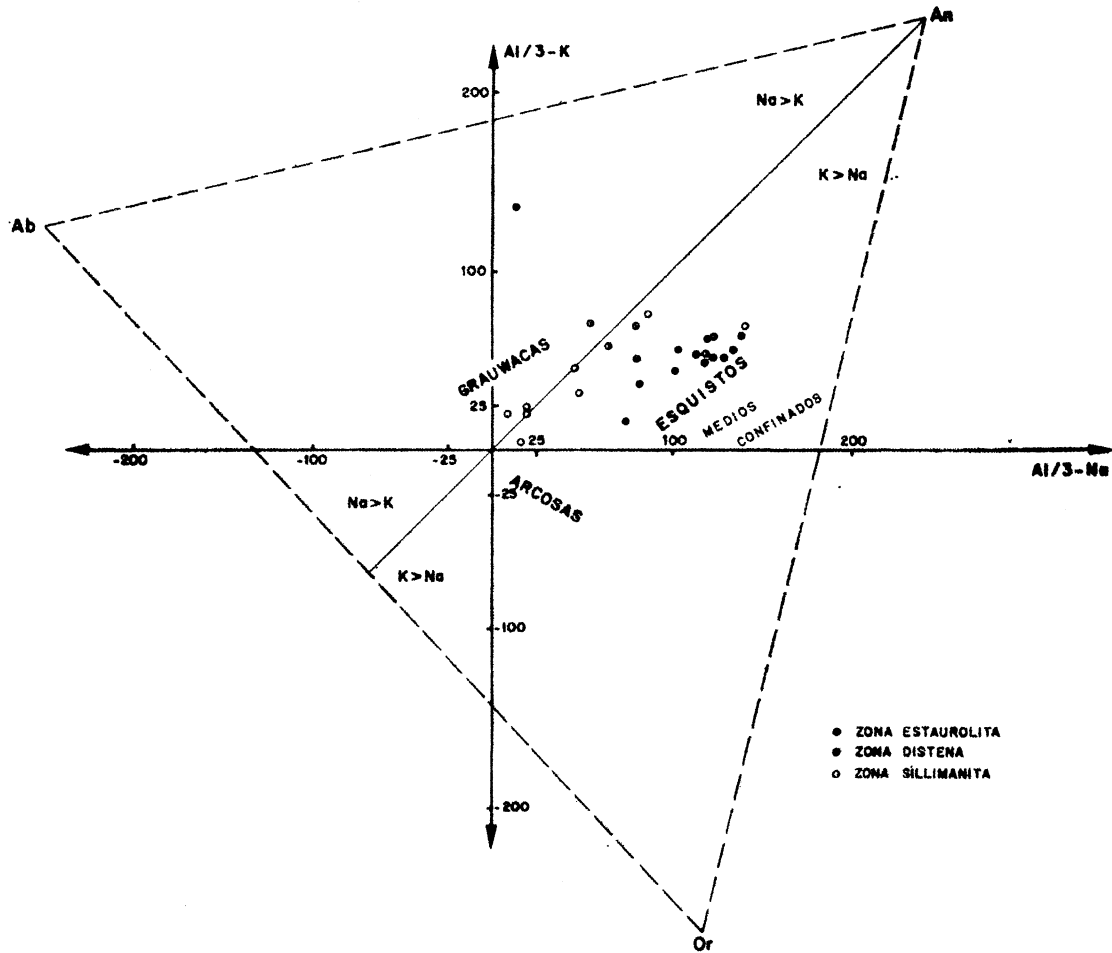
Fig. 3.—Diagrama A1/3 - K — A1/3 - Na de La Roche (1968) para muestras de las zonas de la estauroлита, distena y sillimanita
