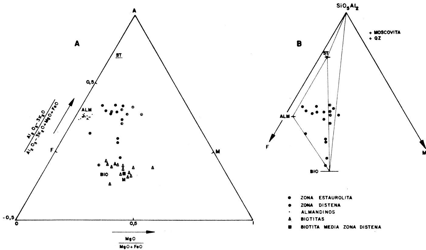
Fig. 5.—Diagrama AFM de Thompson (1957) para las rocas de las zonas de la estaurolita y de la distena
