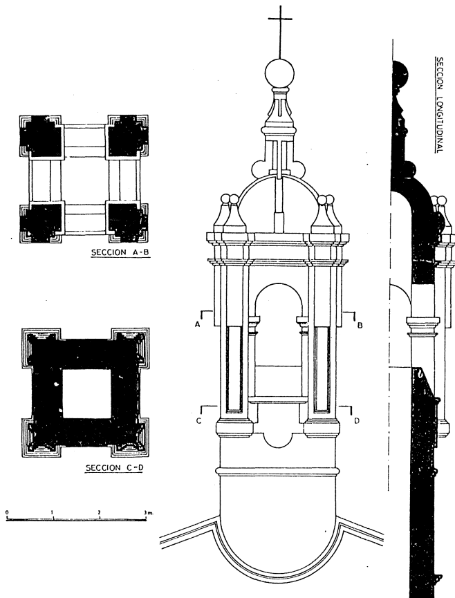
Análisis de la torre.
