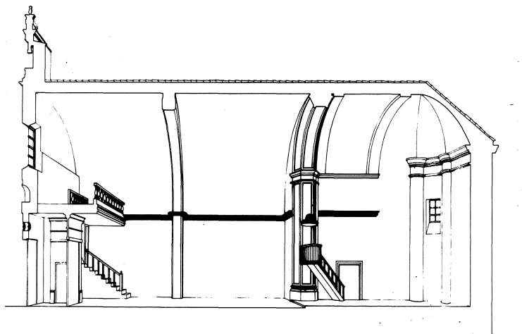
Sección del templo.
