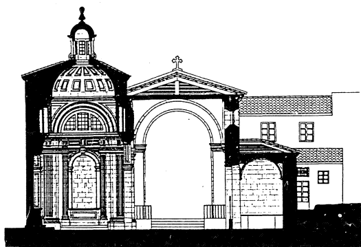
Sección transversal.
