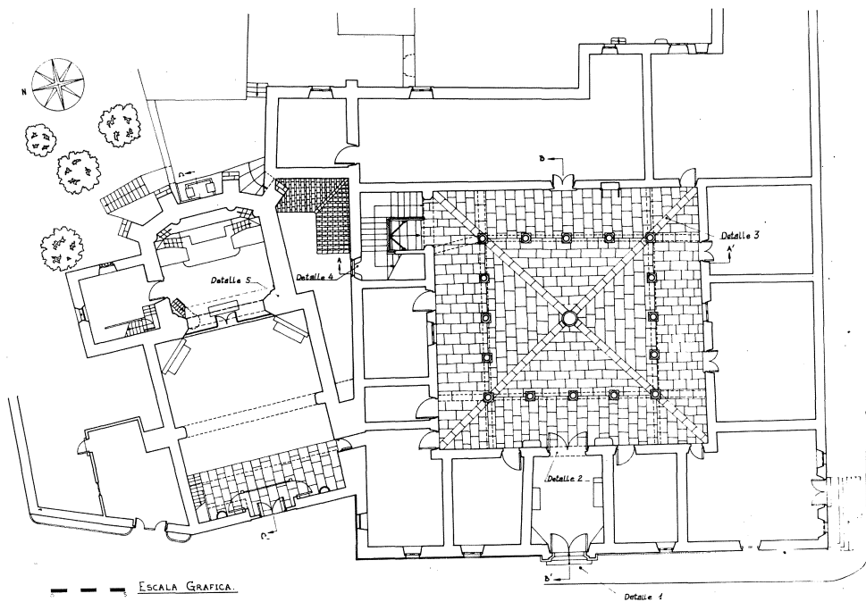
Planta general.
