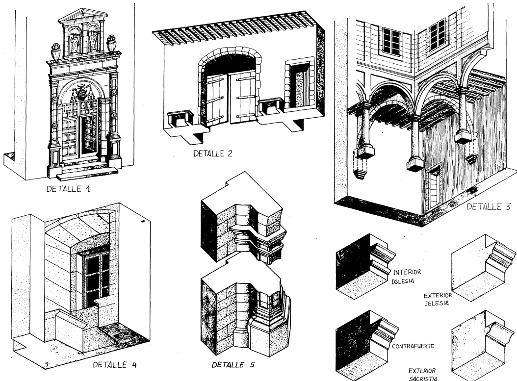
Análisis de los detalles arquitectónicos y constructivos.
