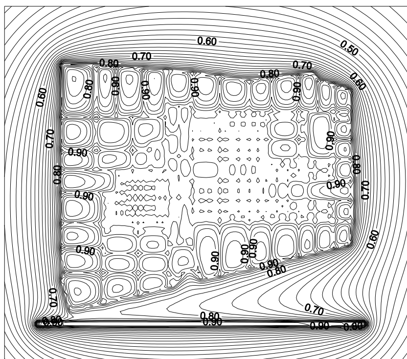
Figura 5. Caso 3: Distribución de potencial ( \times 10 kV) en la superficie del terreno.
