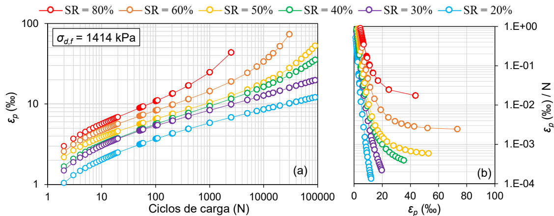
Figura 39 – Resultados de los ensayos RLPDTx de la CRM 2.5B_2.75W, tras 3 días de curado a 50 °C, a los diferentes SR considerados: (a) deformación permanente acumulada frente a número de ciclos de carga; (b) tasa de deformación permanente acumulada frente a la deformación permanente acumulada
