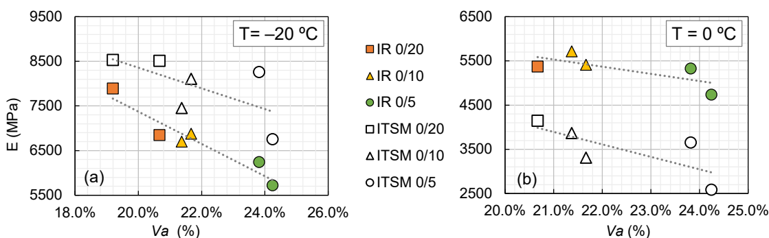
Figura 24 – Comparación entre resultados de ITSM y de módulo dinámico IR a (a) -20 \text{ }^\circ\text{C} , y (b) 0 \text{ }^\circ\text{C} , obtenidos para las mismas probetas de CRM compactadas con método Marshall
