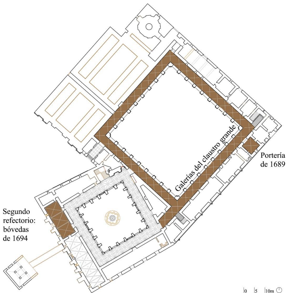
Fig. 1. Planta baja del monasterio de San Julián de Samos señalando las bóvedas de arista construidas entre finales del siglo XVII y mediados del XVIII sobre las galerías del claustro grande, la portería antigua y el segundo refectorio o refectorio de los criados. Dibujo de la autora
