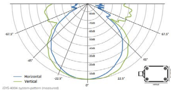
Figura 2. Diagrama de radiación del ISYS-4004.
