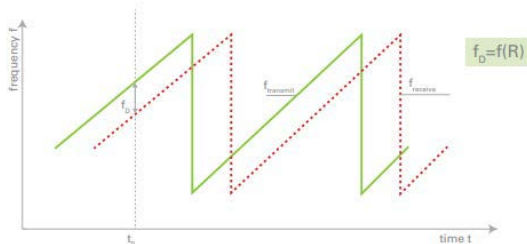
Figura 1. Señal transmitida y recibida en el radar FCMW con modulación diente de sierra.
