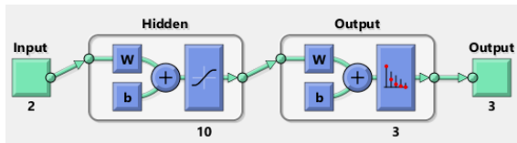
Figura 4. Red neuronal utilizada para la identificación.
