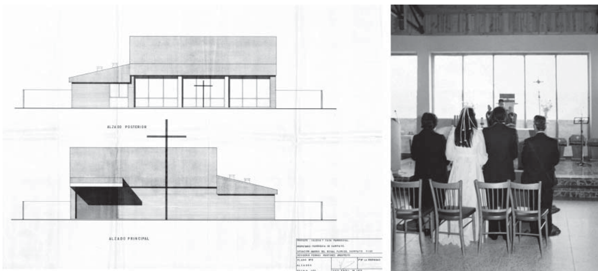
Fig. 25. Desiderio Pernas Martínez. Centro parroquial Sampaio de Lavadores, Vigo (Pontevedra), 1972.
