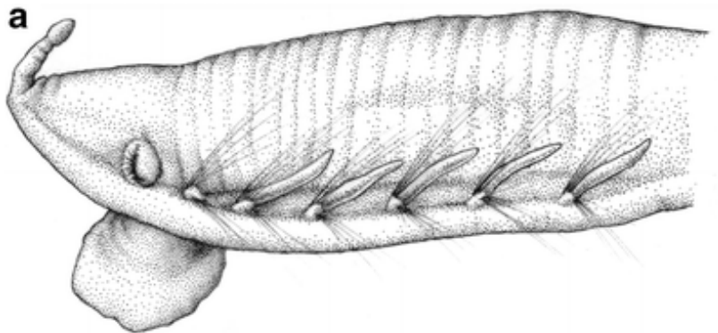
Fig. 5 Ophelina basicirra sp. nov. (holotype, IMNH 24314). a Anterior end, lateral view. b Posterior end, lateral view. Scale bar: 0.5 mm
