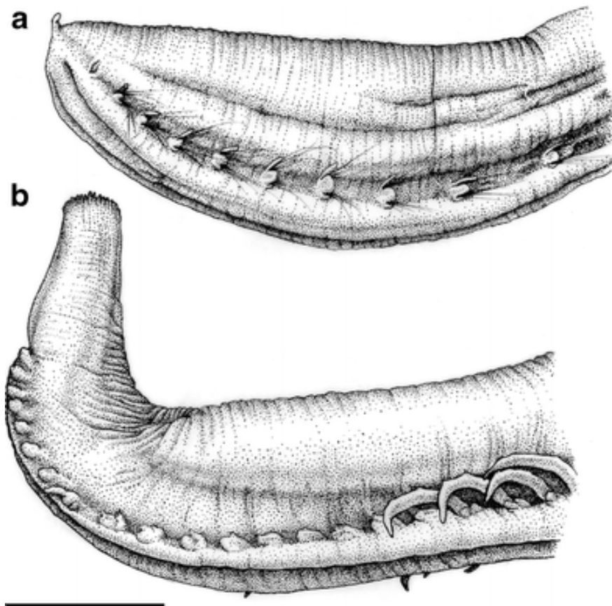
Fig. 12 Ophelina bowitzi sp. nov. (holotype, IMNH 24320).
