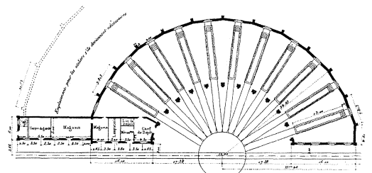
Fig. 352. Remise demi-circulaire pour deux machines. — Compagnie d'Orléans. — Remise de Vendôme. Plan. — Échelle de 0-000 par mètre.
