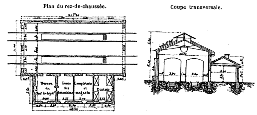
Fig. 347. — Remise pour deux locomotives. Compagnie d'Orléans
