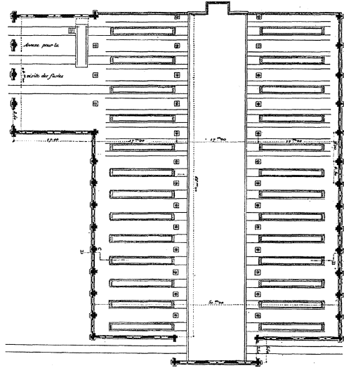
Fig. 355. — Remise rectangulaire pour machines. — Compagnie d'Orléans. — Remise de Périgueux. — Plan. — Échelle de 0 m ,002 par mètre.
