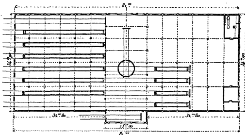
Fig. 355. Remise rectangulaire de Bar-le-Duc.
