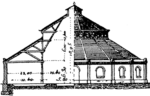
Fig. 188. Remise polygonale. Coupe et élévation.
