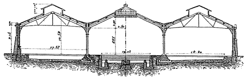
Fig. 352. -- Remise de Montargis. -- Coupe transversale. -- Echelle de 0,002 par mètre.
