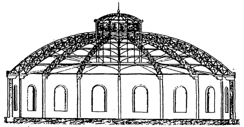
Fig. 212. -- Remise polygonale des Ardennes.
