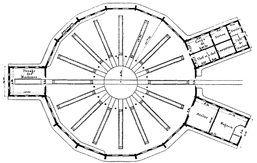
Fig. 351. -- Remise circulaire de locomotive. Compagnie P.-L.-M. -- Remise de Montargis. -- Plan. -- Echelle de 0,002 par mètre.
