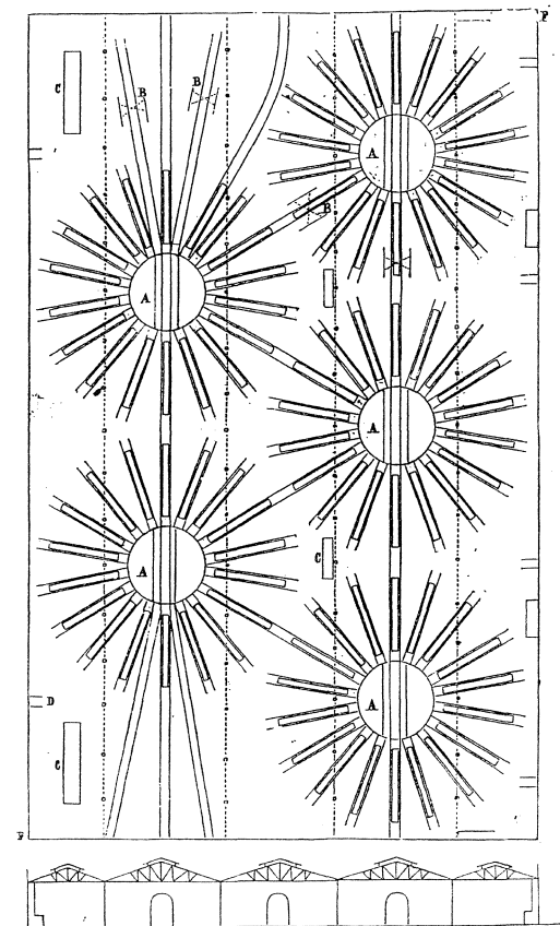
Fig. 214. — Grande remise de Gateshead.
