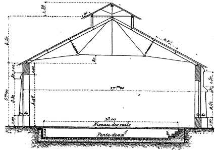
Fig. 354. — Remise de Vendôme. — Coupe transversale. — Échelle de 0-005 par mètre.
