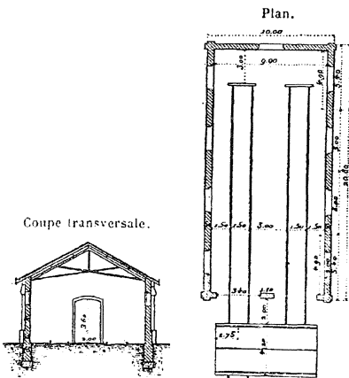
Fig. 346. — Remise pour 4 voitures. — Compagnie
