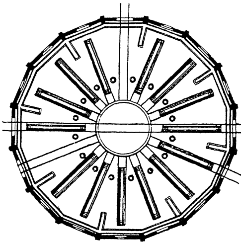
Fig. 189. R-mise polygonale. - Plan.
