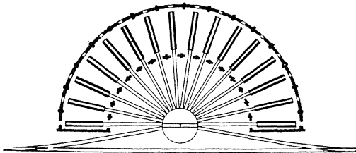
Fig. 191. Remise en fer à cheval. Fig. 273. — Remise en fer à cheval.
