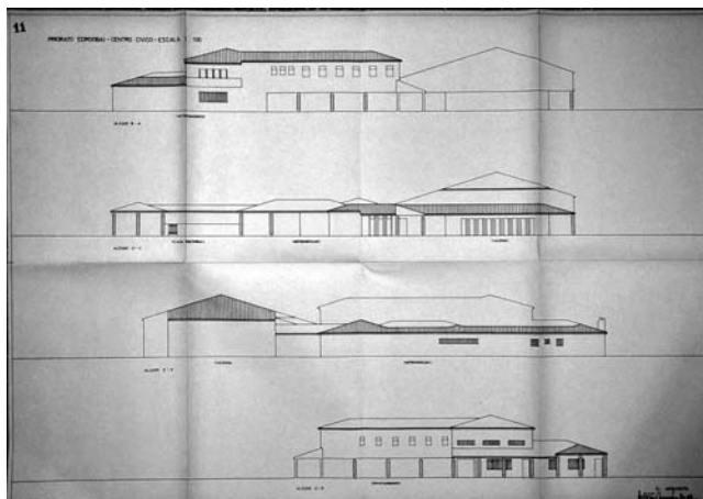
Fig. 06. Antonio Fernández Alba, El Priorato (Córdoba), 1964; alzado presentado en el proyecto inicial sin campanario.
