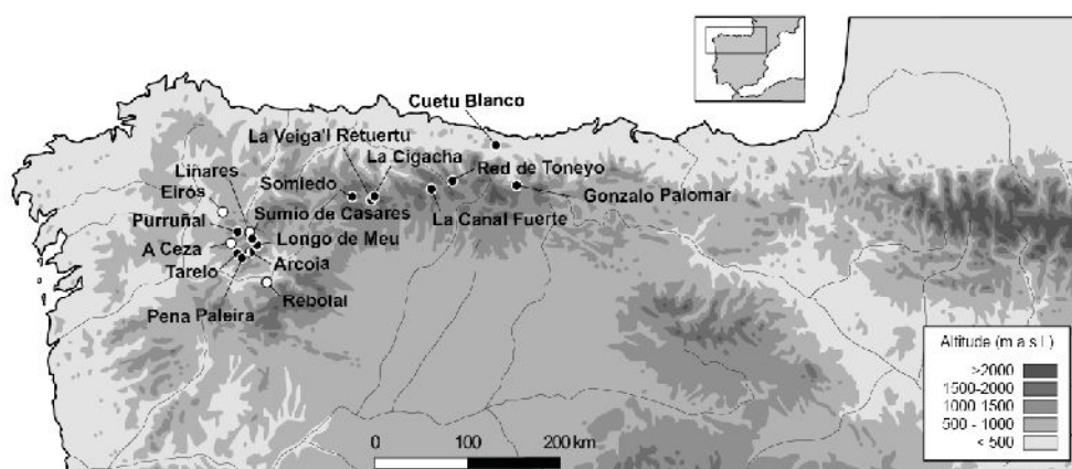
Fig. 1. Mapa de situación de las cuevas estudiadas en el Noroeste de la Península Ibérica. Con círculos blancos se destacan los yacimientos con oso cavernario; los círculos negros muestran los yacimientos con oso pardo.
