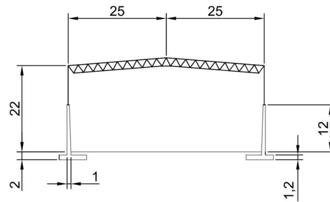
SECCIÓN AA'
