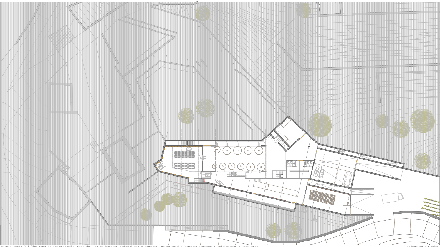
planta corte 225.25m zona de fermentación, cava de vino en barrica, embotellado y cava de vino en botella_zona de almacenaje instalaciones y vestuarios
