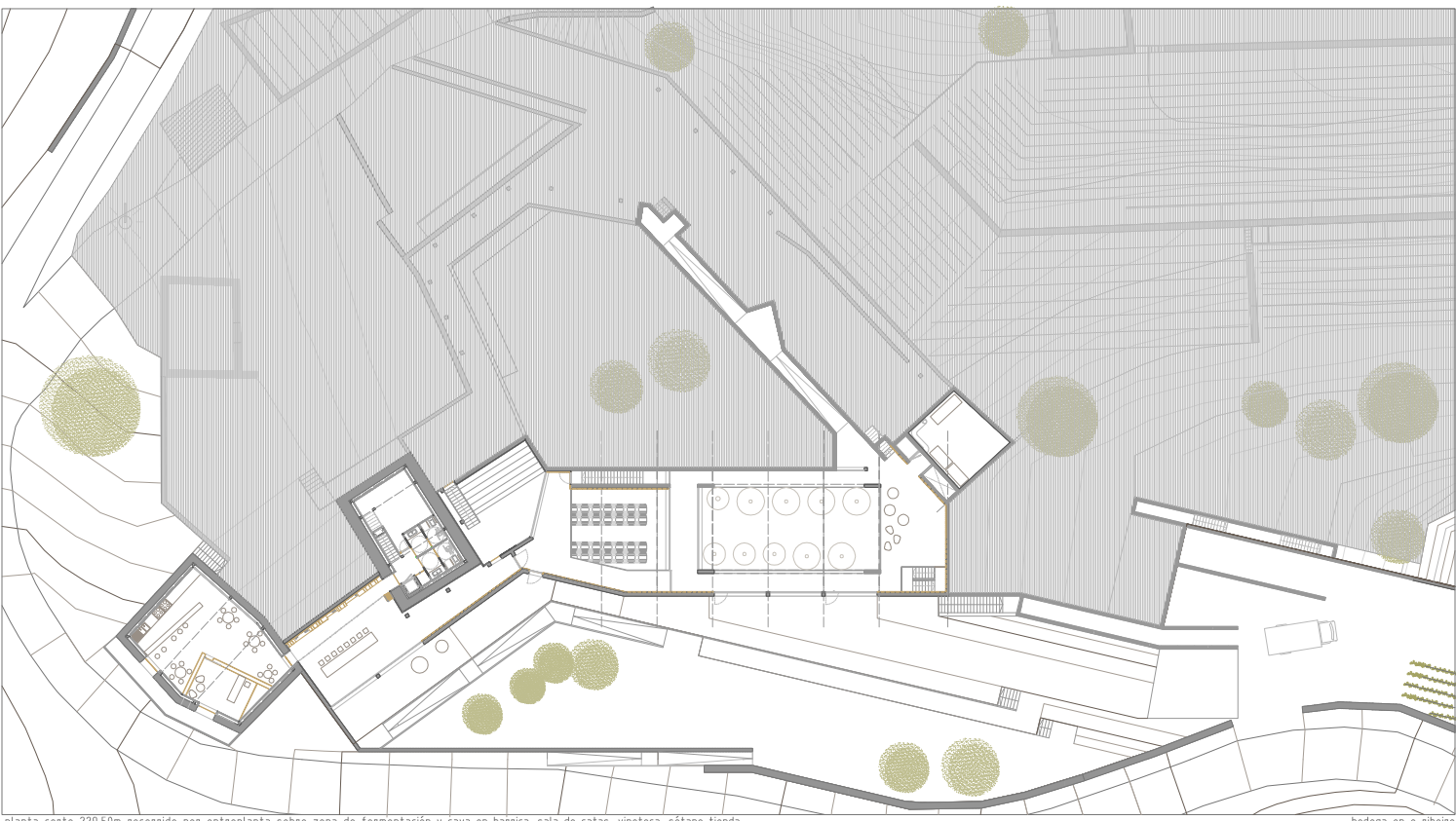
planta corte 229.50m recorrido por entreplanta sobre zona de fermentación y cava en barrica, sala de catas, vinoteca, sótano tienda
