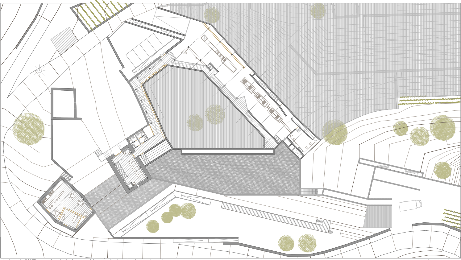
planta corte 233.00m zona de entrada de uva y elaboración_tienda, inicio del recorrido, vinoteca
