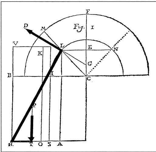
Figura 7 Representación del equilibrio de fuerzas y momentos, con ayuda de una "biela acodada" (basado en La Hire 1712)
