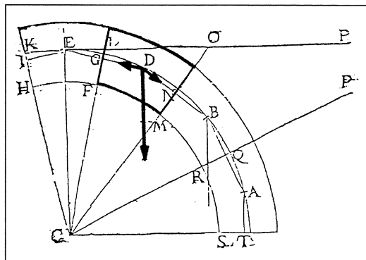
Figura 3 Equilibrio de una dovela
