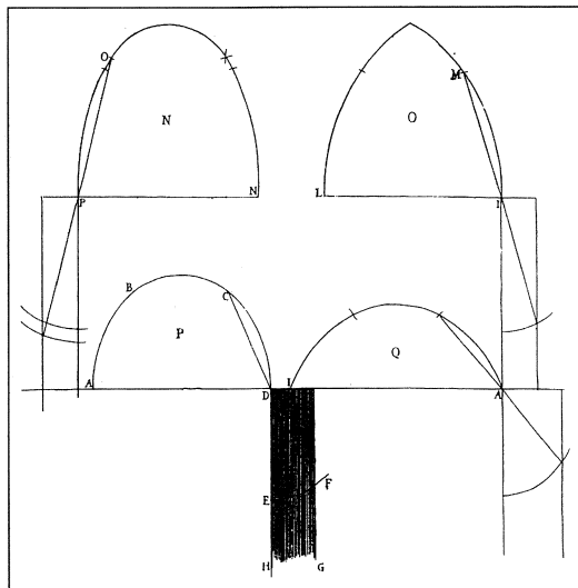
Figura 1 Regla geométrica gótica para el cálculo de los estribos (Derand, 1643)
